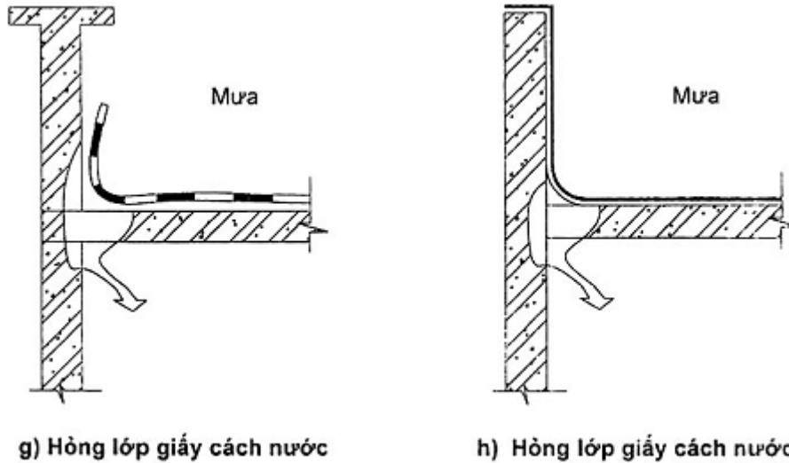
Hình 20 - Các dạng thấm qua mái bê tông cốt thép
