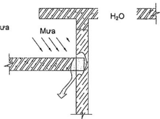
d) Chỗ tiếp giáp mái với cổ tường
